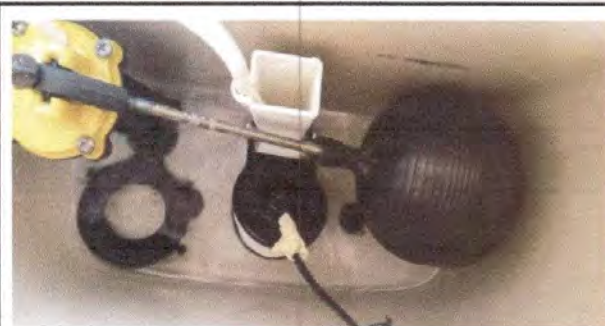
Foto 10: Sustitución de accesorios inodoro (contra llave, tubo de abasto y tanque) módulo dos
